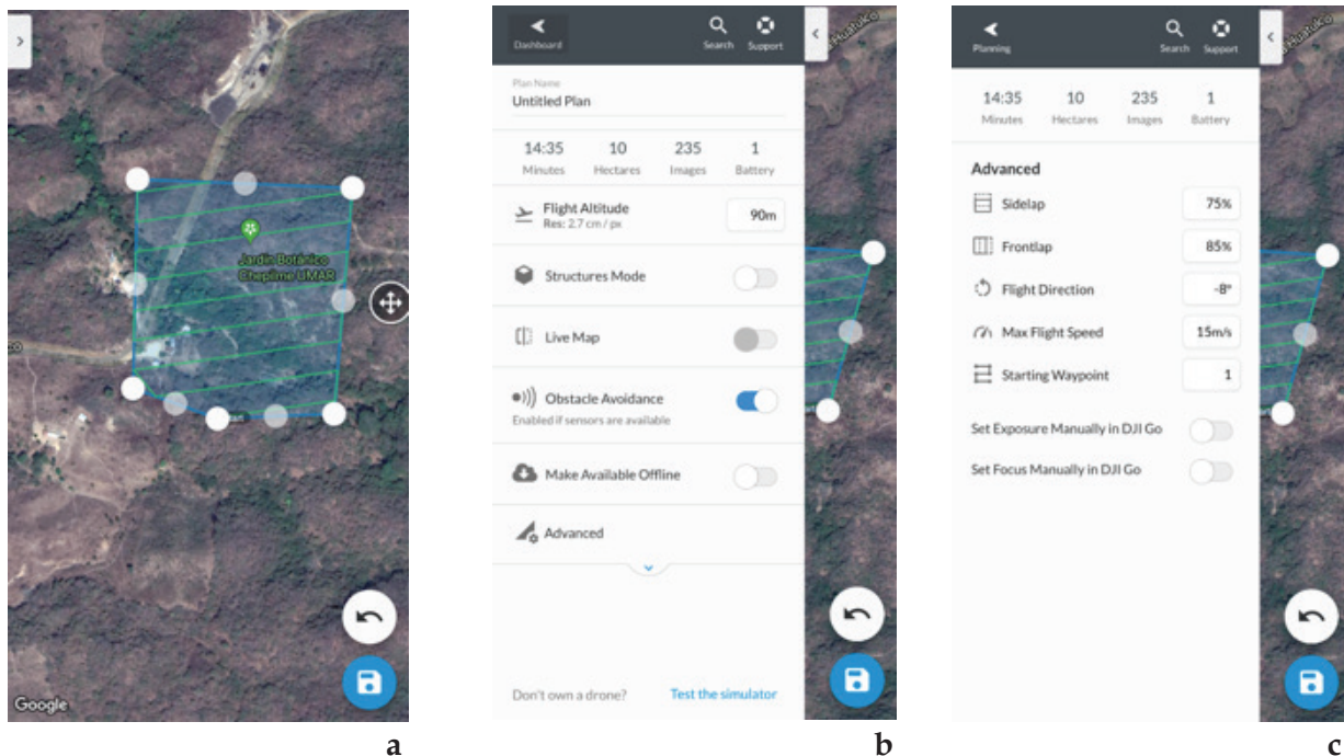
Figura 2. Configuración de plan de vuelo a) Plan de vuelo, b) Configuración de altura de vuelo, tiempo, superficie a cubrir y número de baterías, c) Configuración de sobrelape, velocidad, dirección de vuelo e inicio de vuelo.
